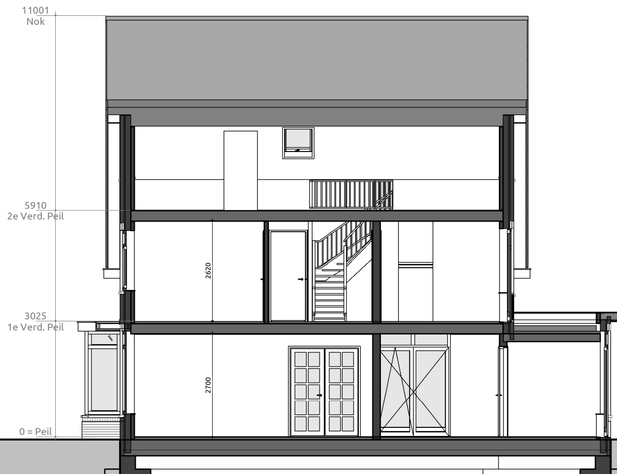
Doorsnede A - A
