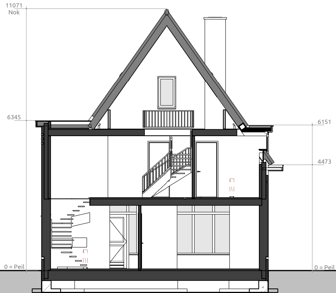
Doorsnede B - B
