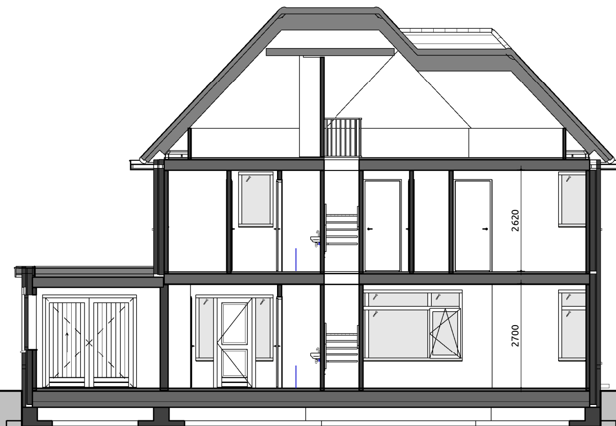
Doorsnede B - B
