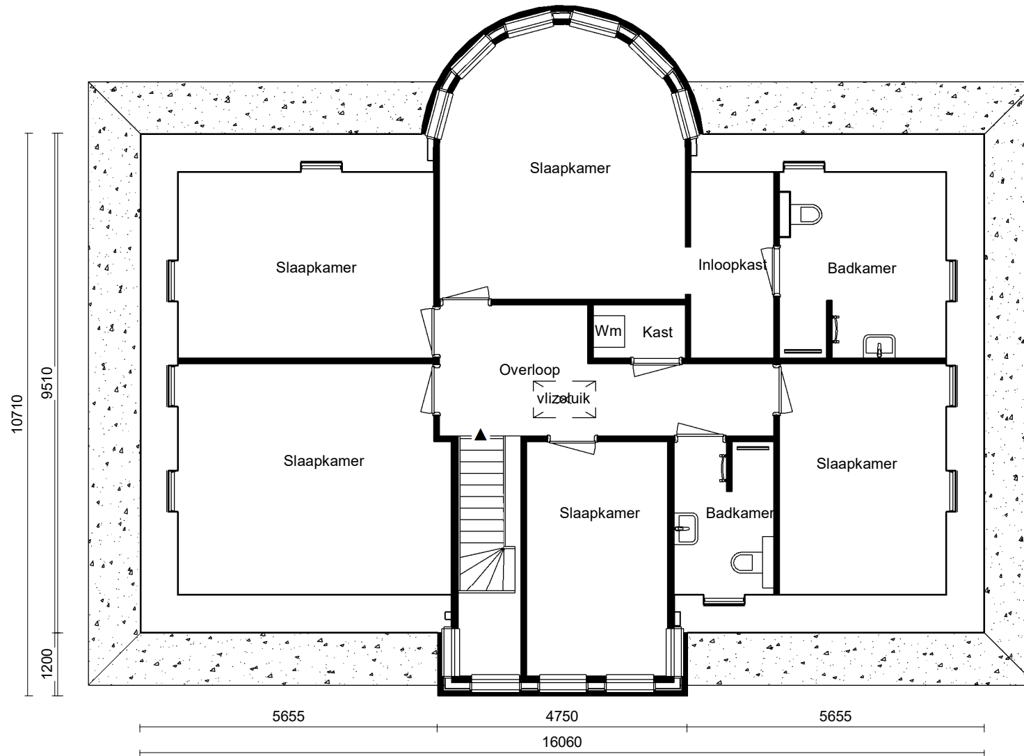
Eerste verdieping
