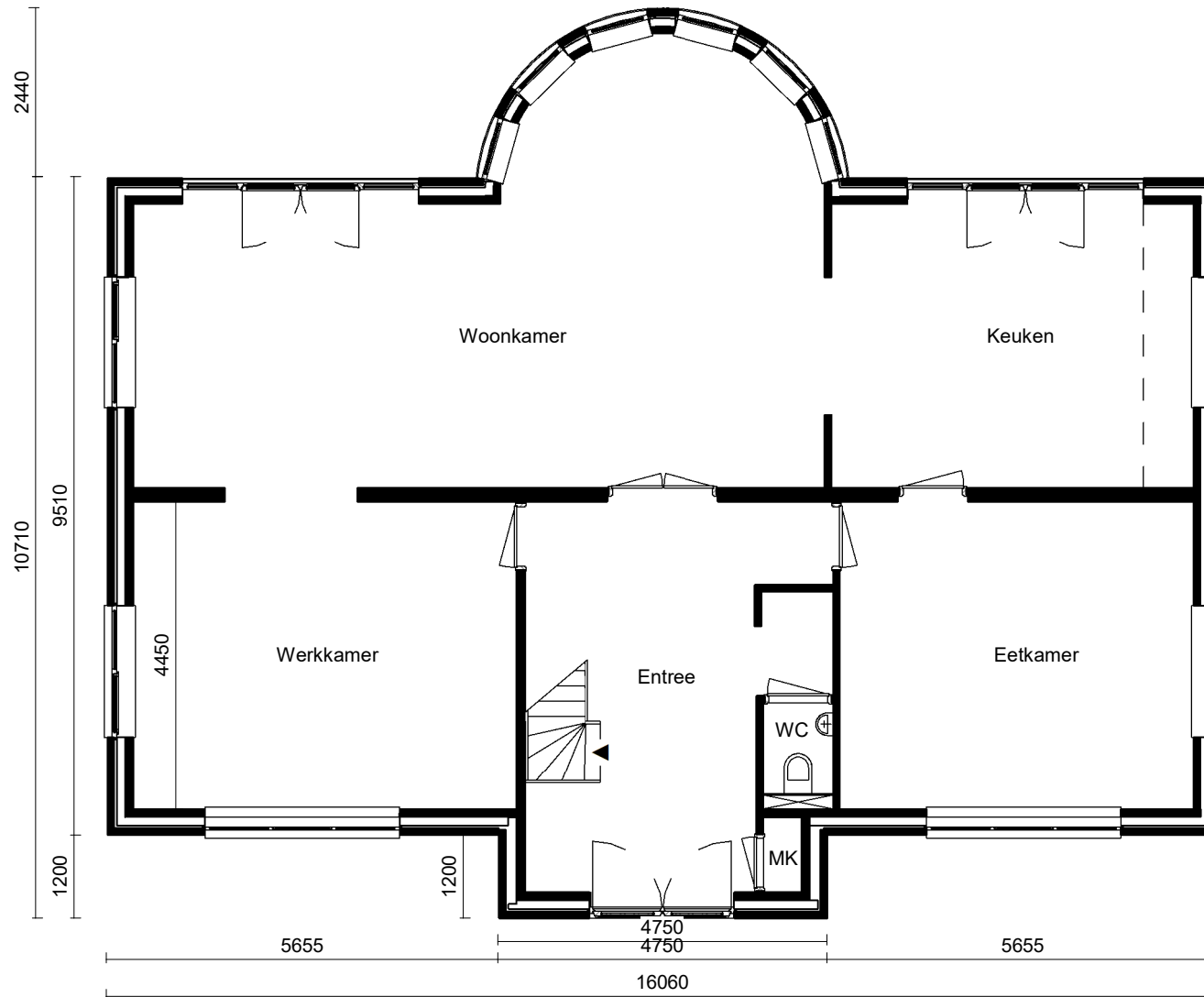
Begane grond
