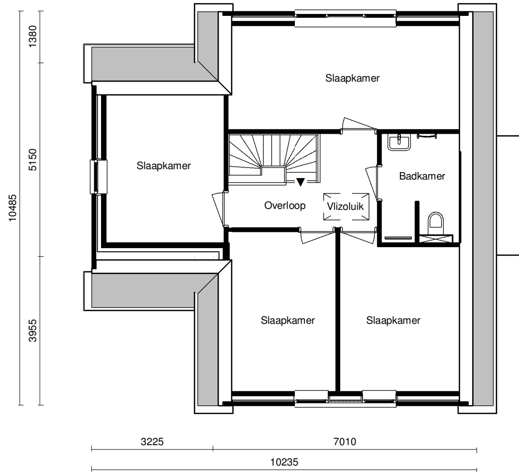
Eerste verdieping
