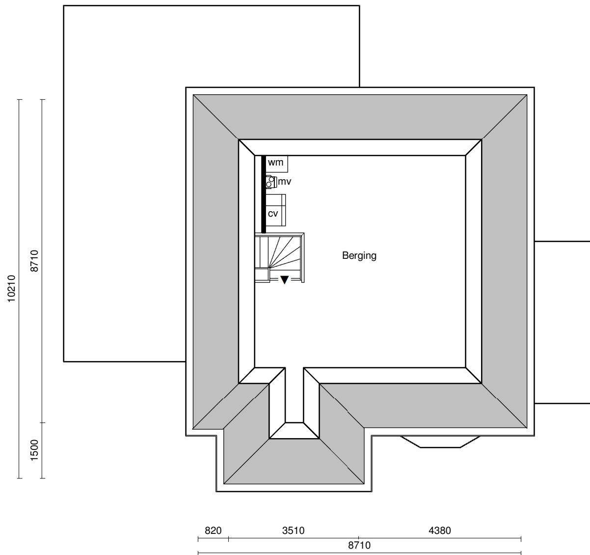
Tweede verdieping
