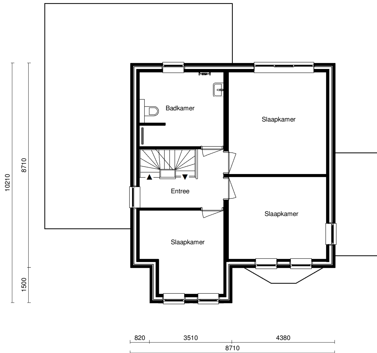
Eerste verdieping
