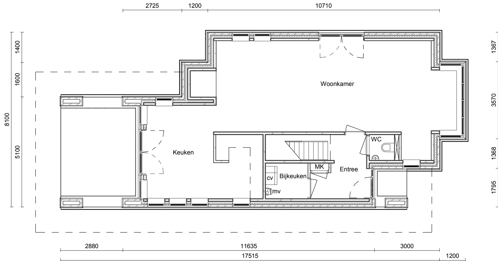
Begane grond
