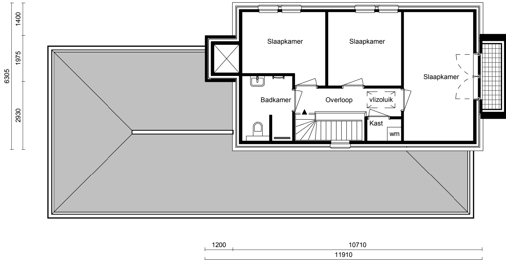
Eerste verdieping
