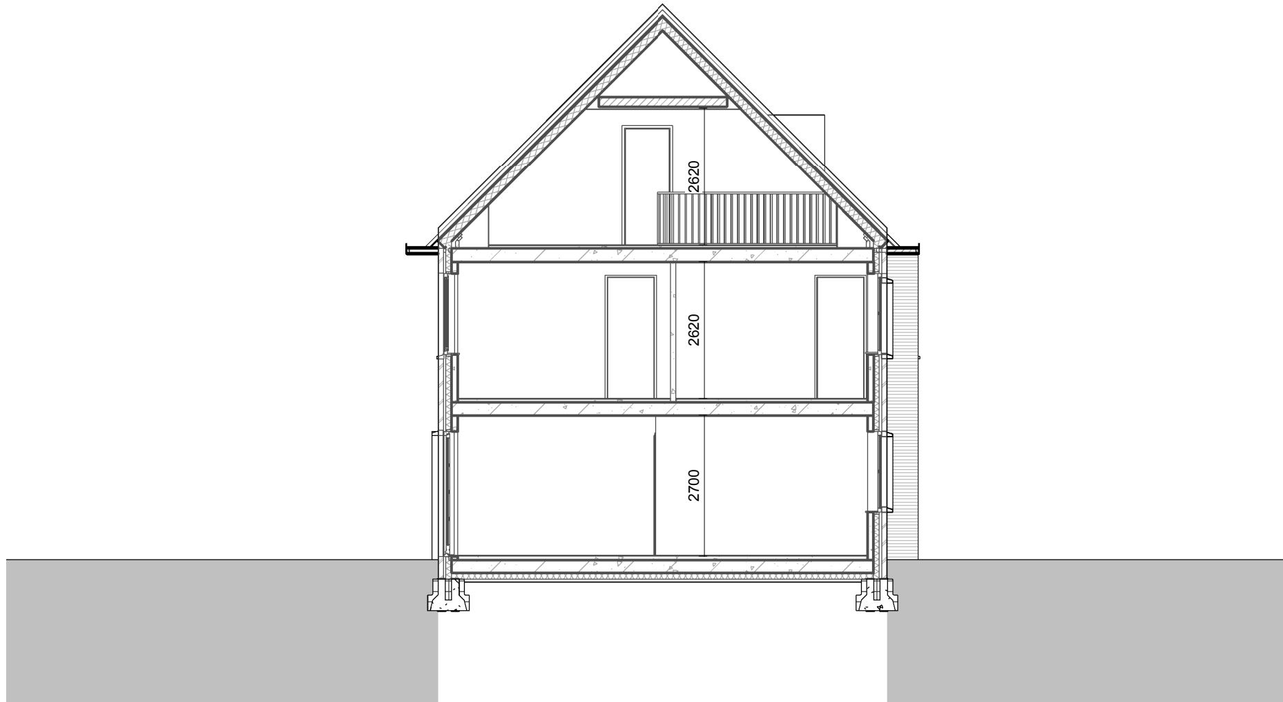
Doorsnede A-A
