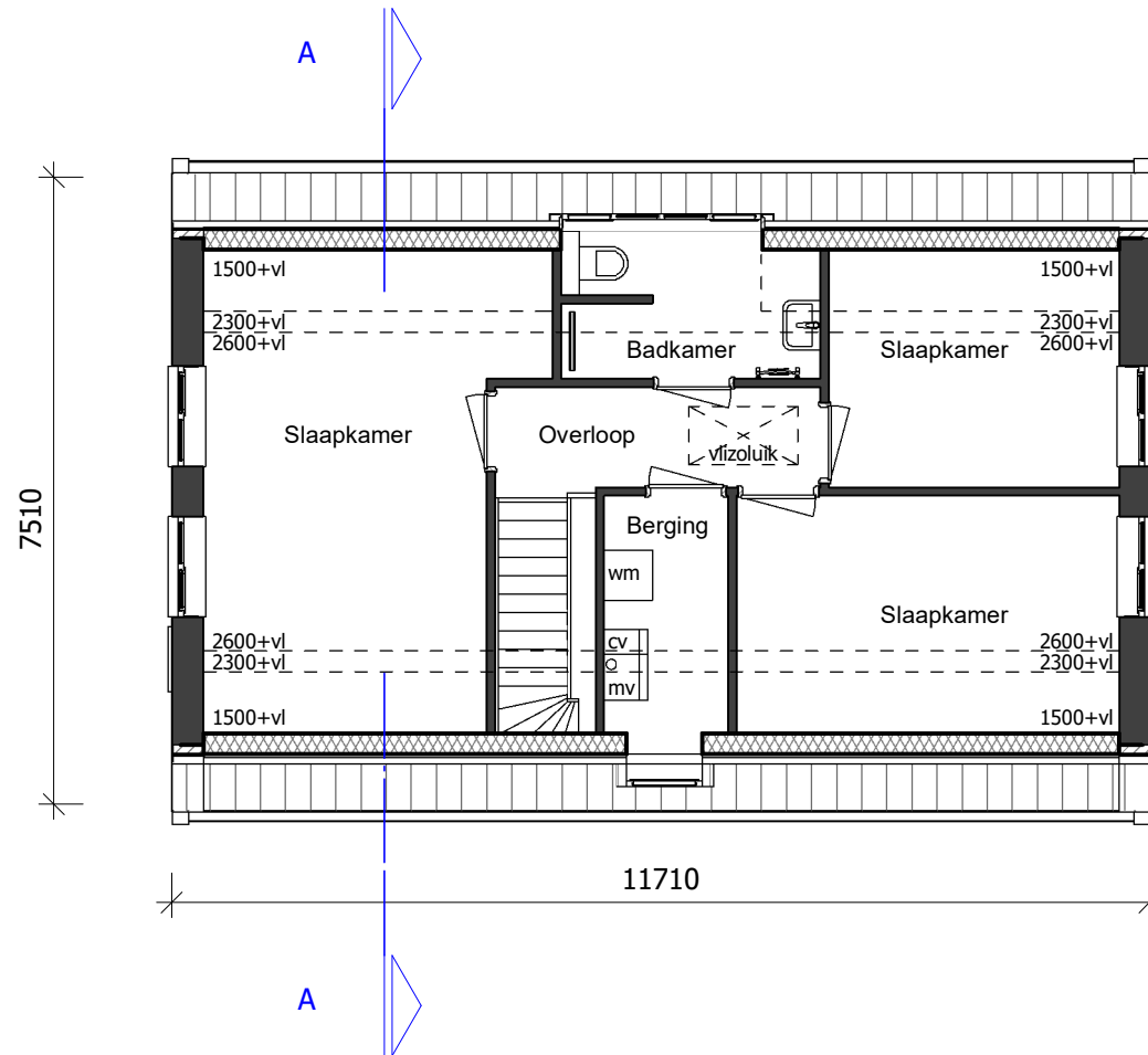
Eerste verdieping
