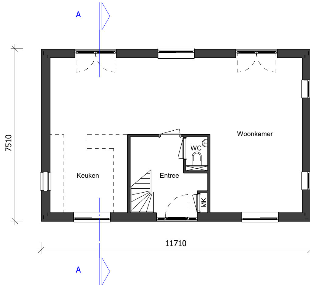
Begane grond
