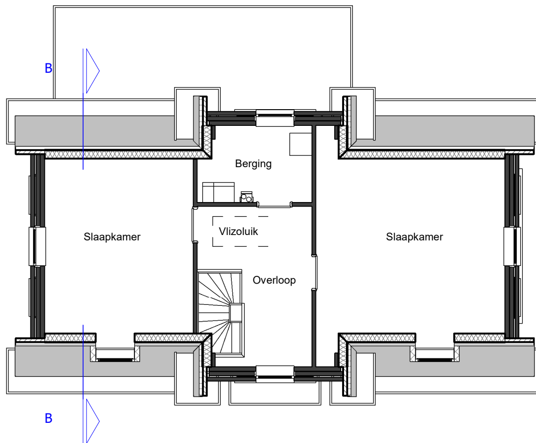
Tweede verdieping
