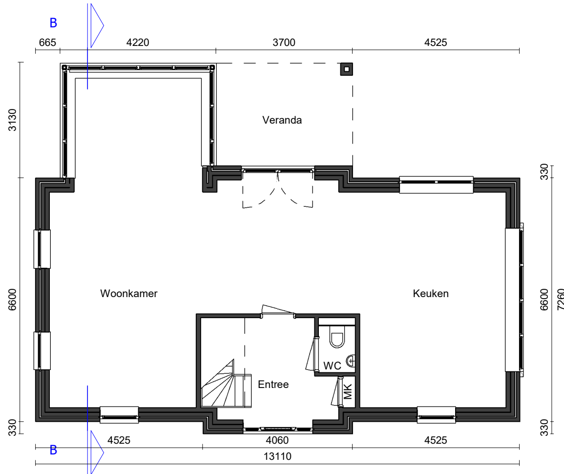
Begane grond
