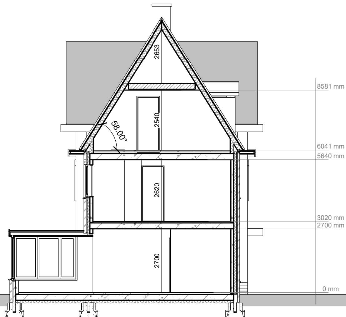
Doorsnede B - B
