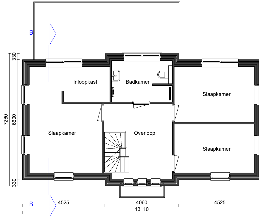
Eerste verdieping
