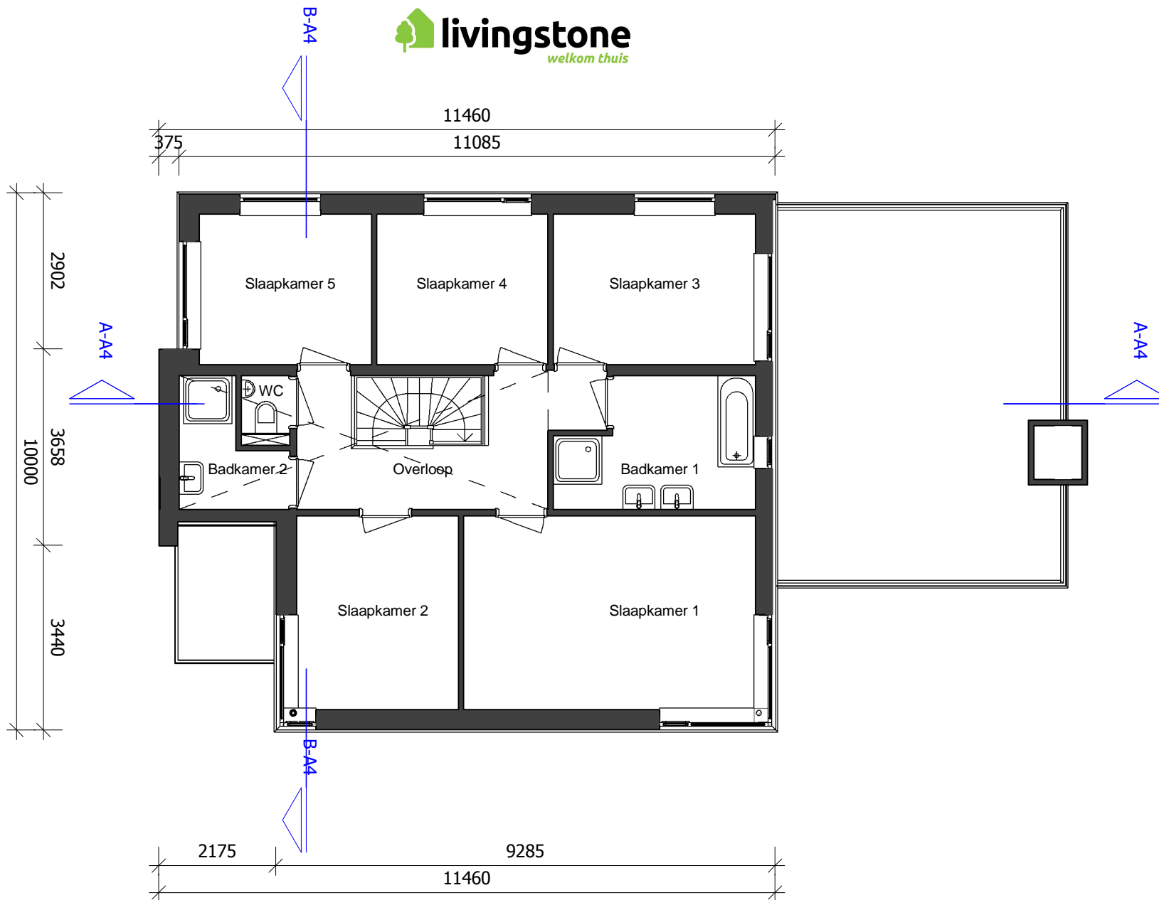
Eerste verdieping
