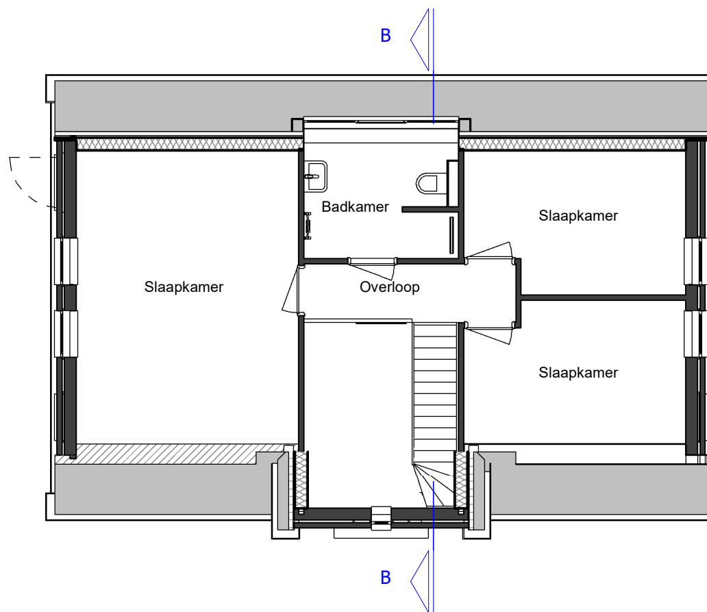
Eerste verdieping
