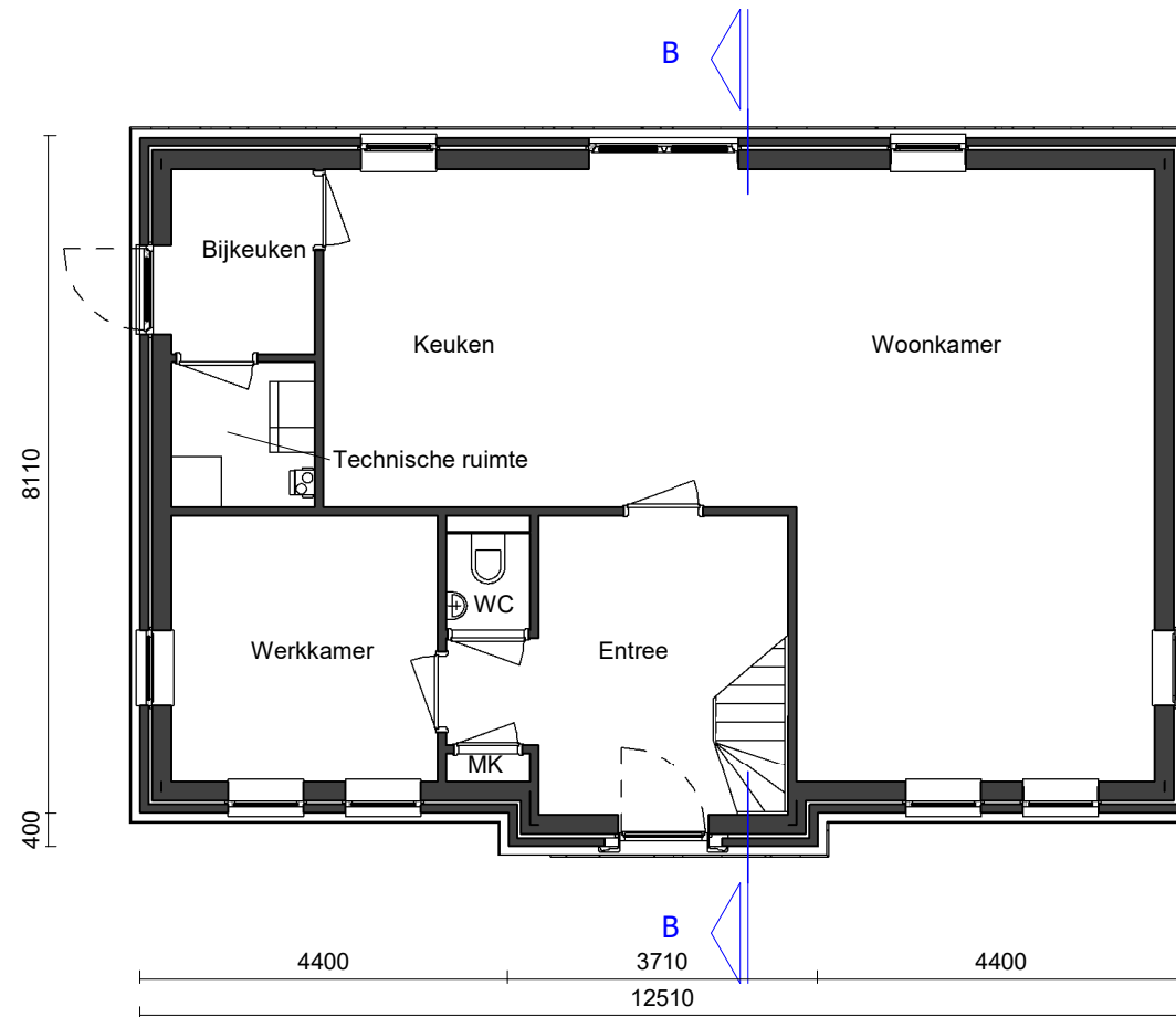
Begane grond
